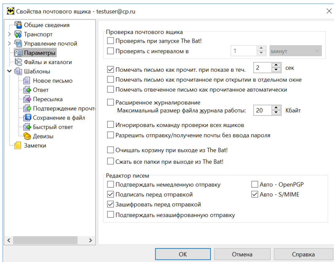
Рисунок 116. Редактирование свойств почтового ящика
