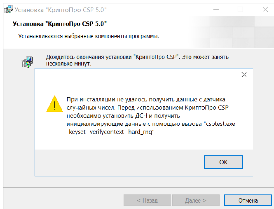
Рисунок 12. Окно ошибки получения данных с ДСЧ
