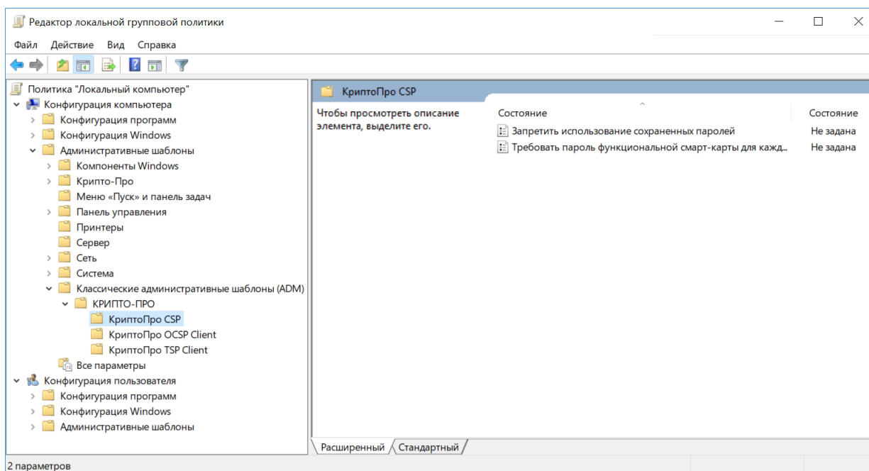
Рисунок 157. Параметры групповой политики для СКЗИ КриптоПро CSP
