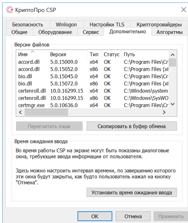
Рисунок 78. Вкладка Дополнительно панели управления
