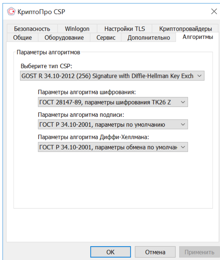
Рисунок 80. Вкладка Алгоритмы панели управления
