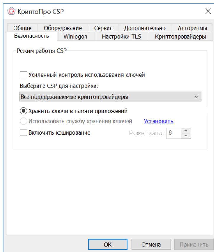
Рисунок 77. Установка службы хранения ключей
