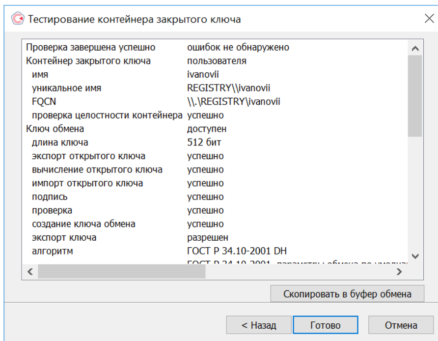
Рисунок 51. Окно с результатами тестирования контейнера
